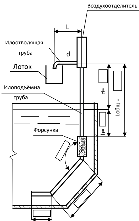
Схема эрлифта А
