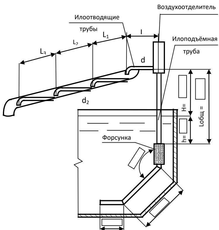
Схема эрлифта Б
